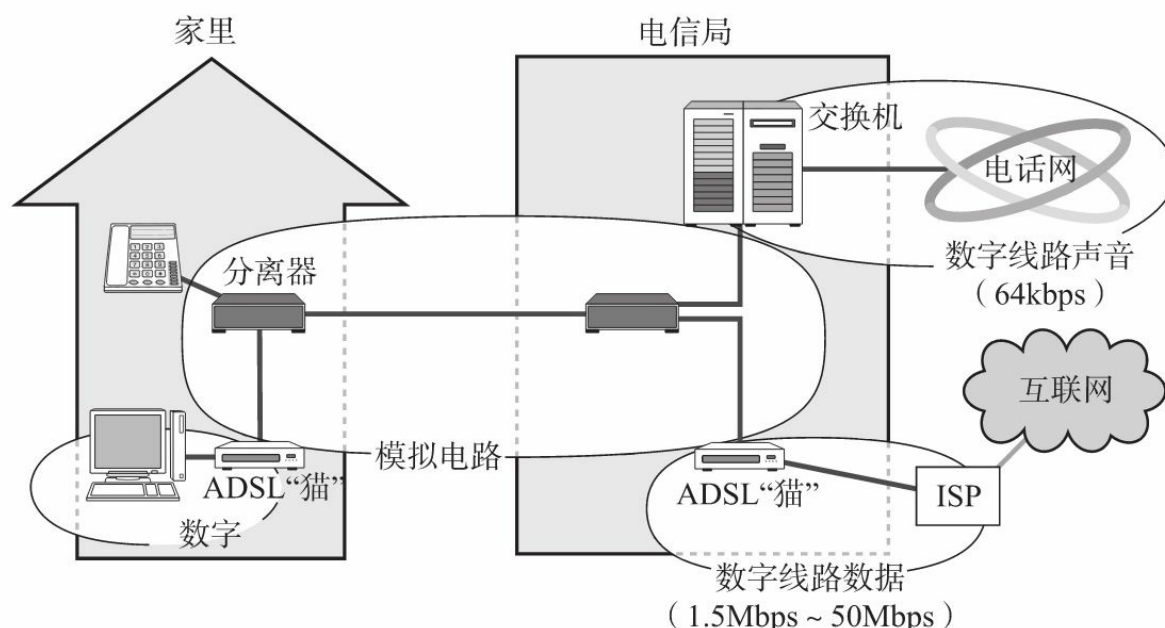
图3.34 ADSL连接
