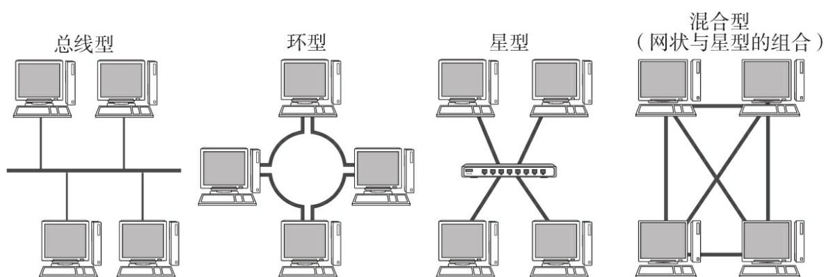
图3.3 总线型、环型、星型、网状型
