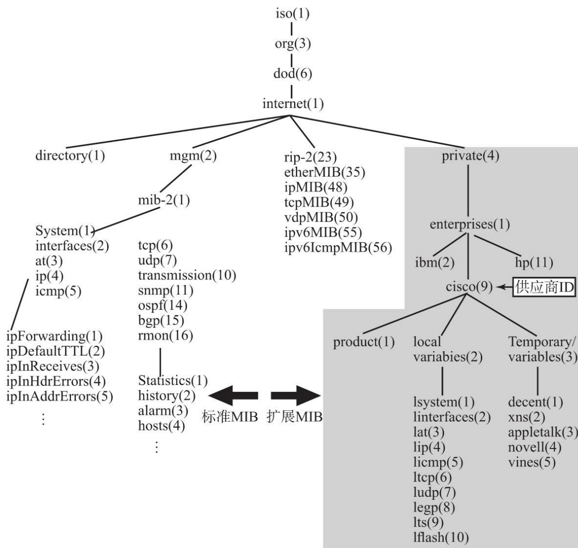
图8.22 MIB树举例（Cisco Systems相关）
