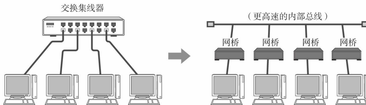
图1.43 交换集线器是网桥的一种
