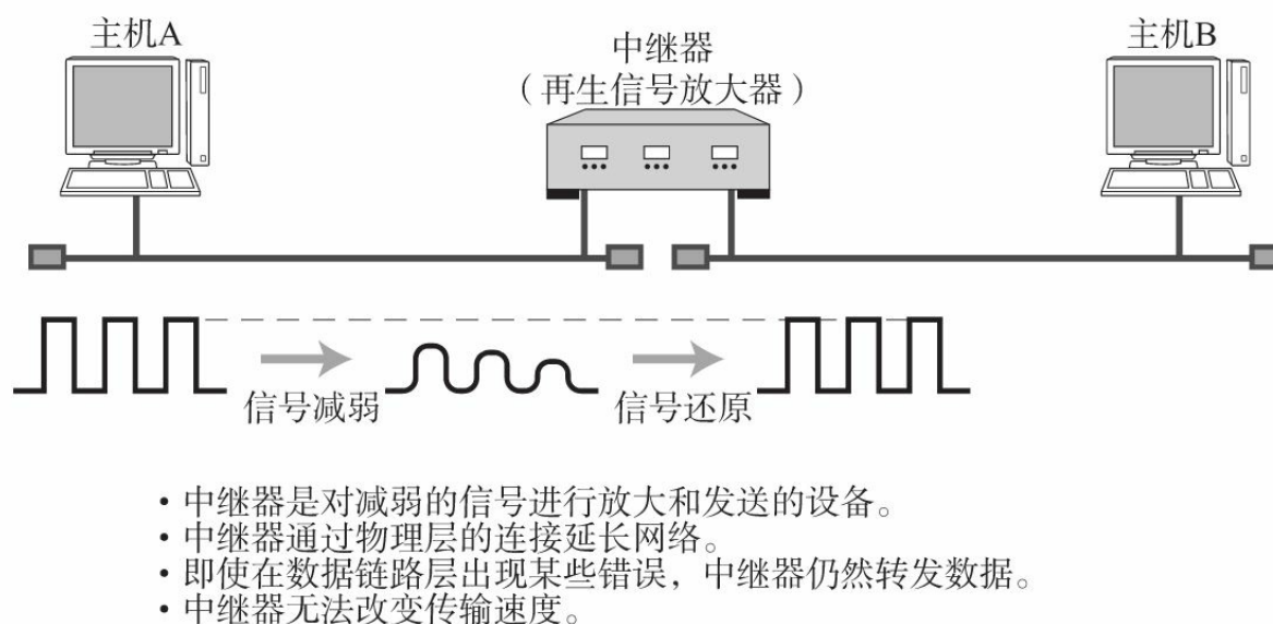
图1.39 中继器
