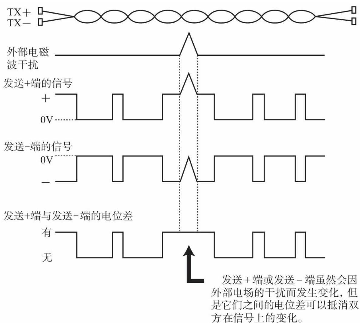
附图.8 双绞线的信号传输方式
