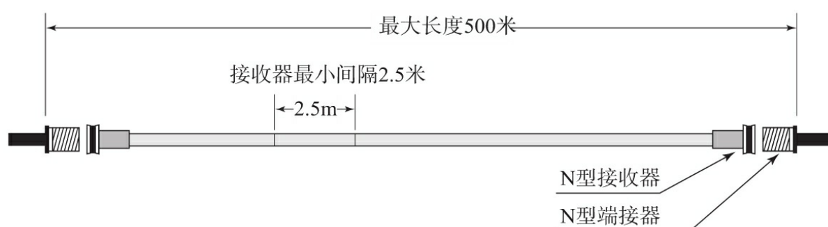
附图.5 以太网电缆（10BASE5）
