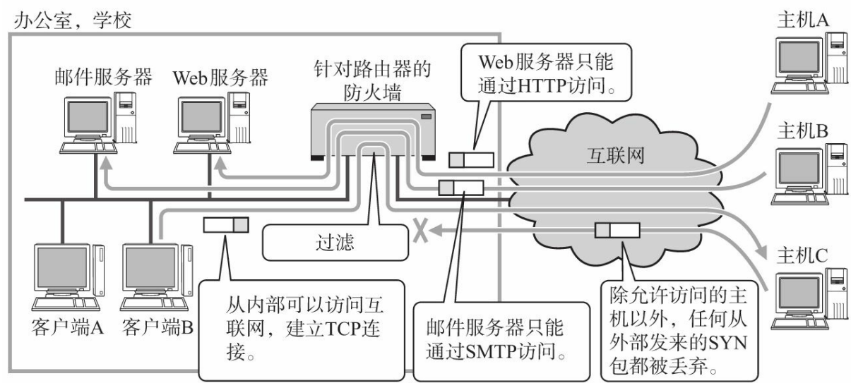
图9.2 防火墙举例
