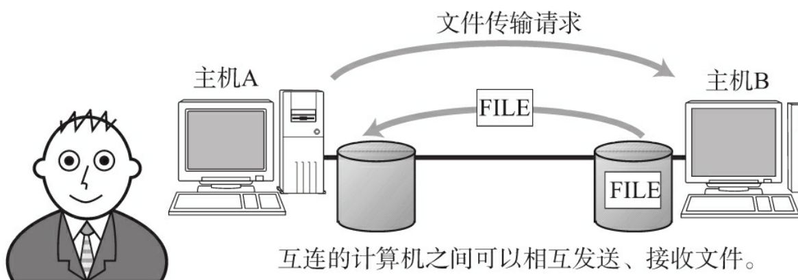
图2.14 FTP
