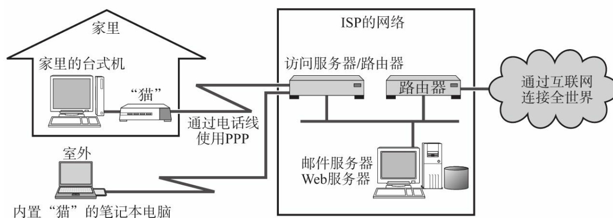
图3.33 拨号连接
