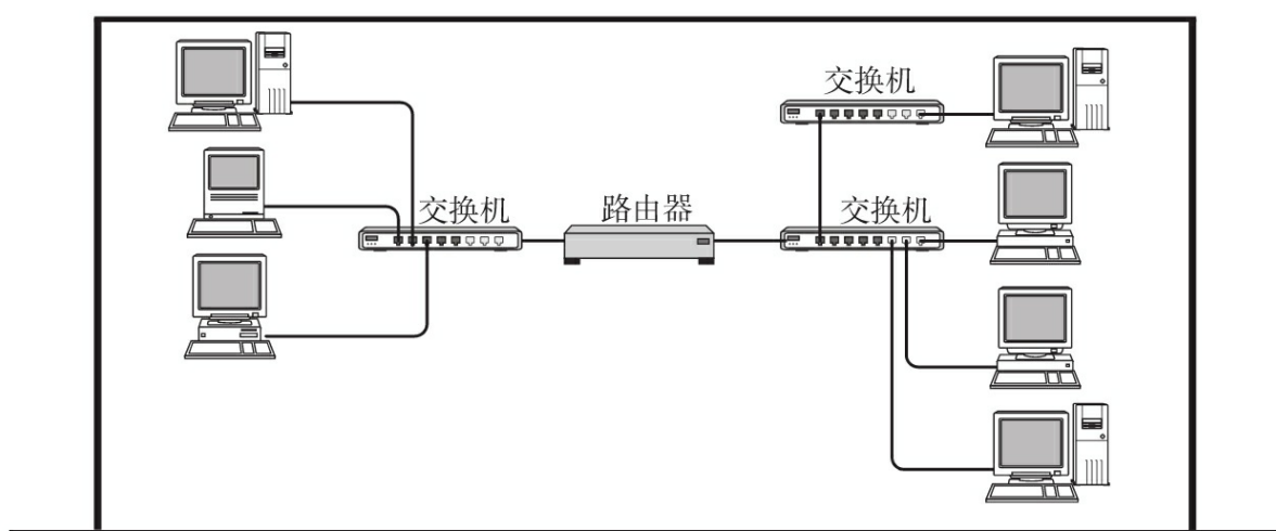
图1.3 LAN
