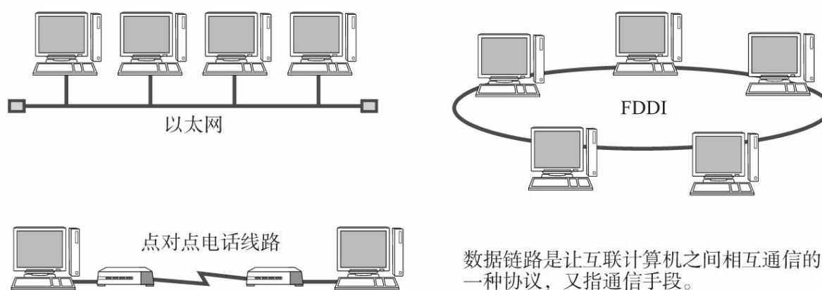
图3.1 数据链路
