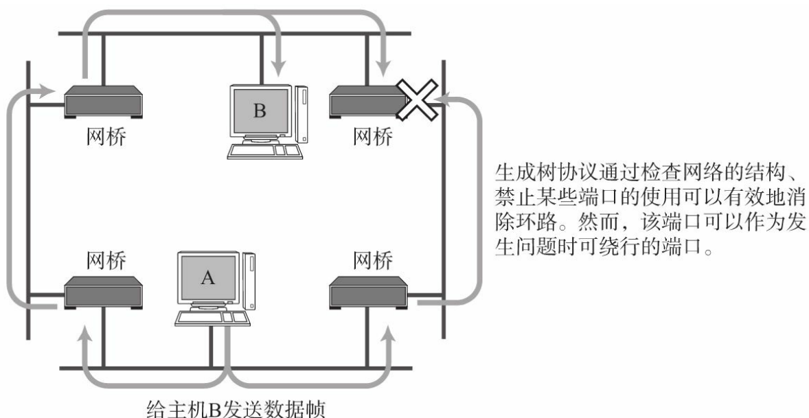
图3.14 生成树法
