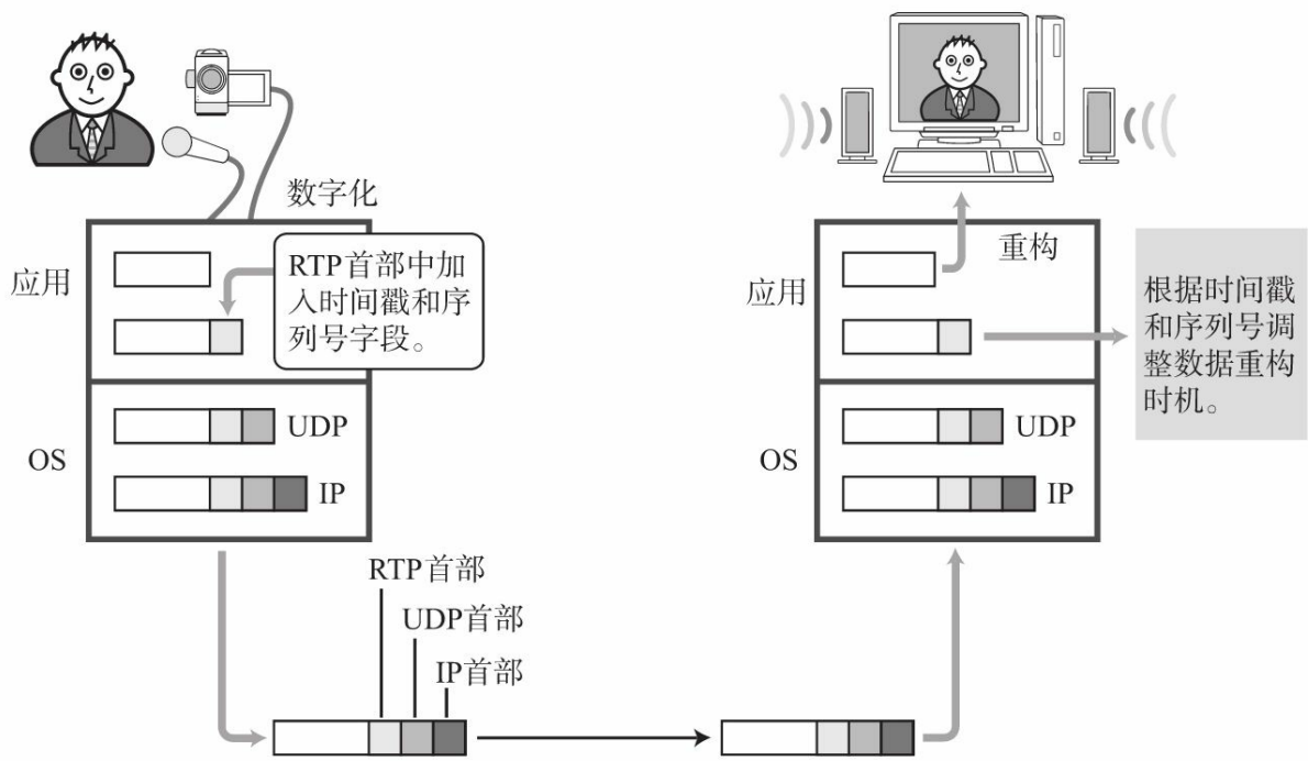
图8.27 RTP通信
