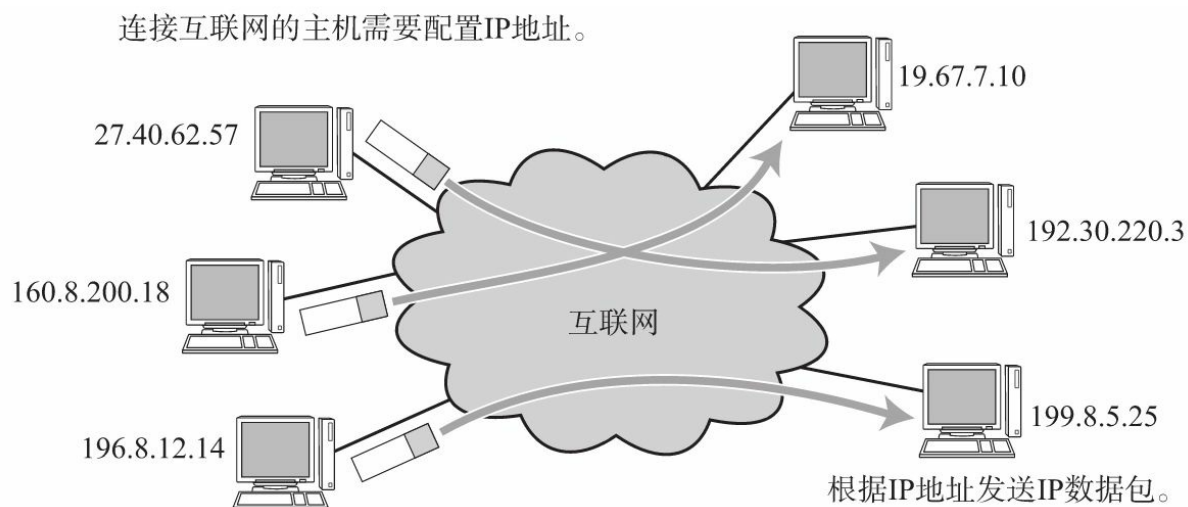
图4.3 IP地址
