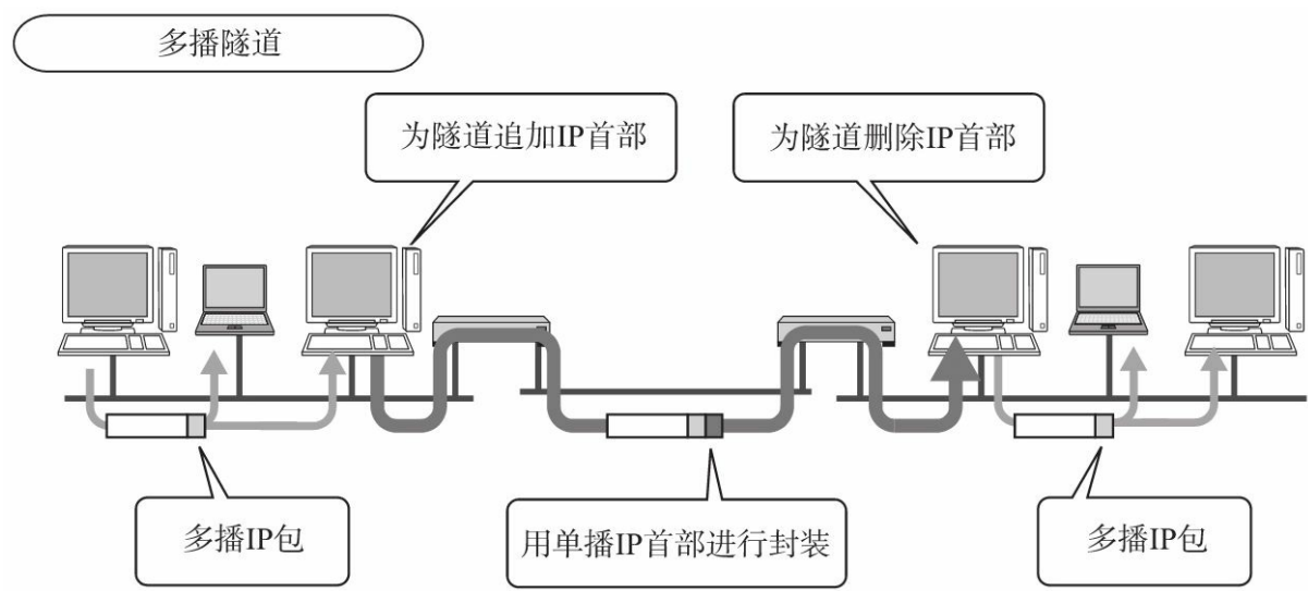
图5.24 多播隧道
