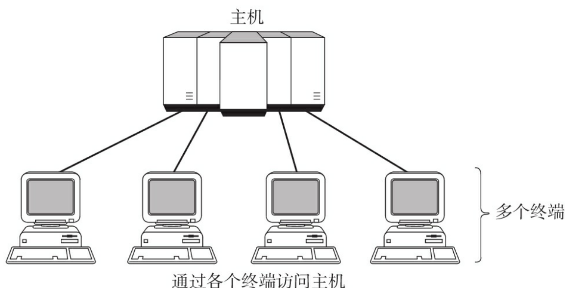
图1.6 分时系统
