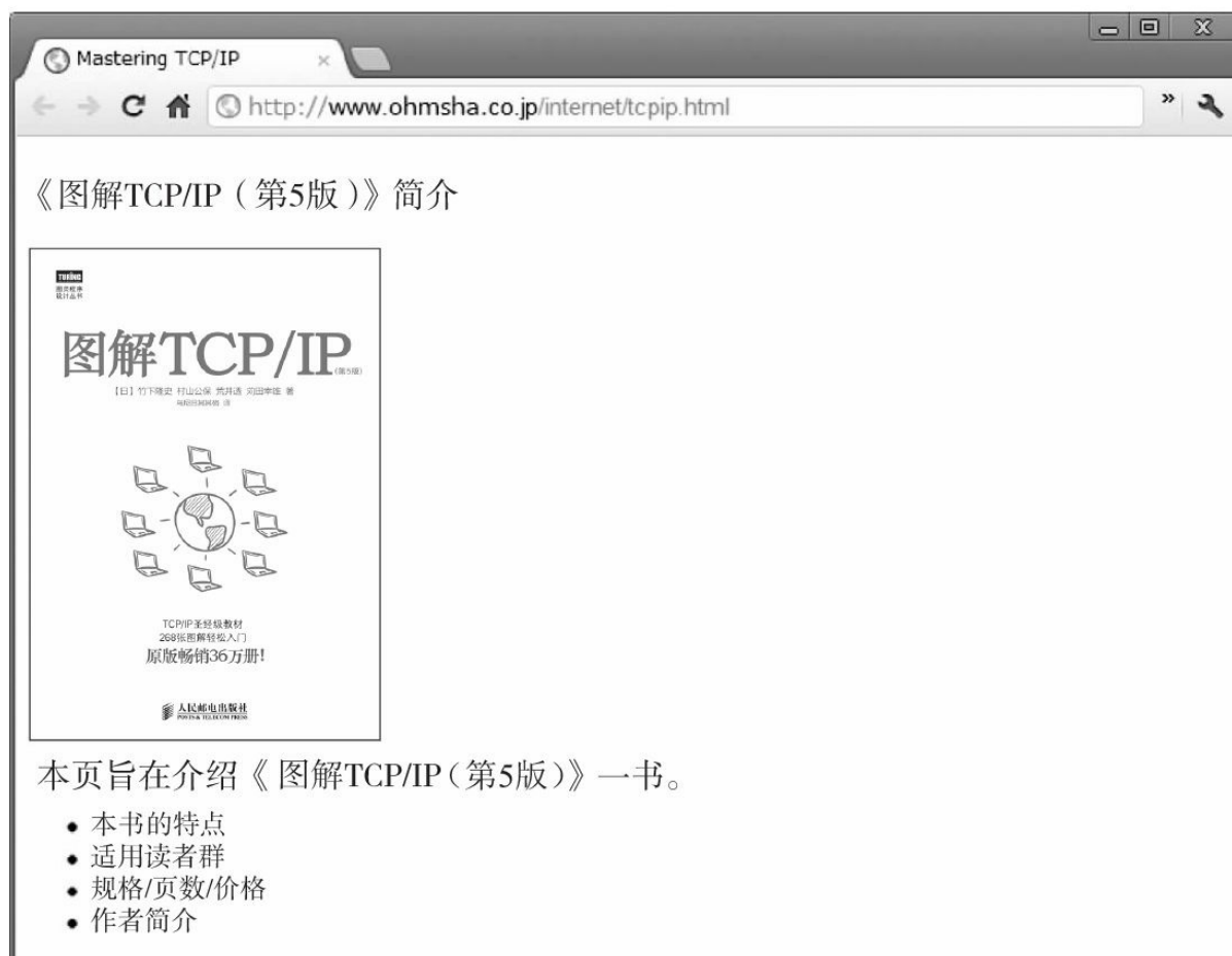
图8.16 HTML举例
