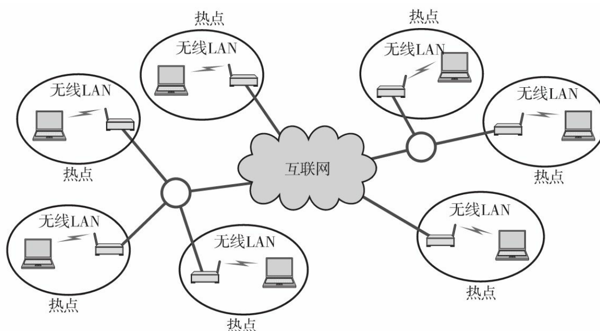
图3.38 无线LAN
