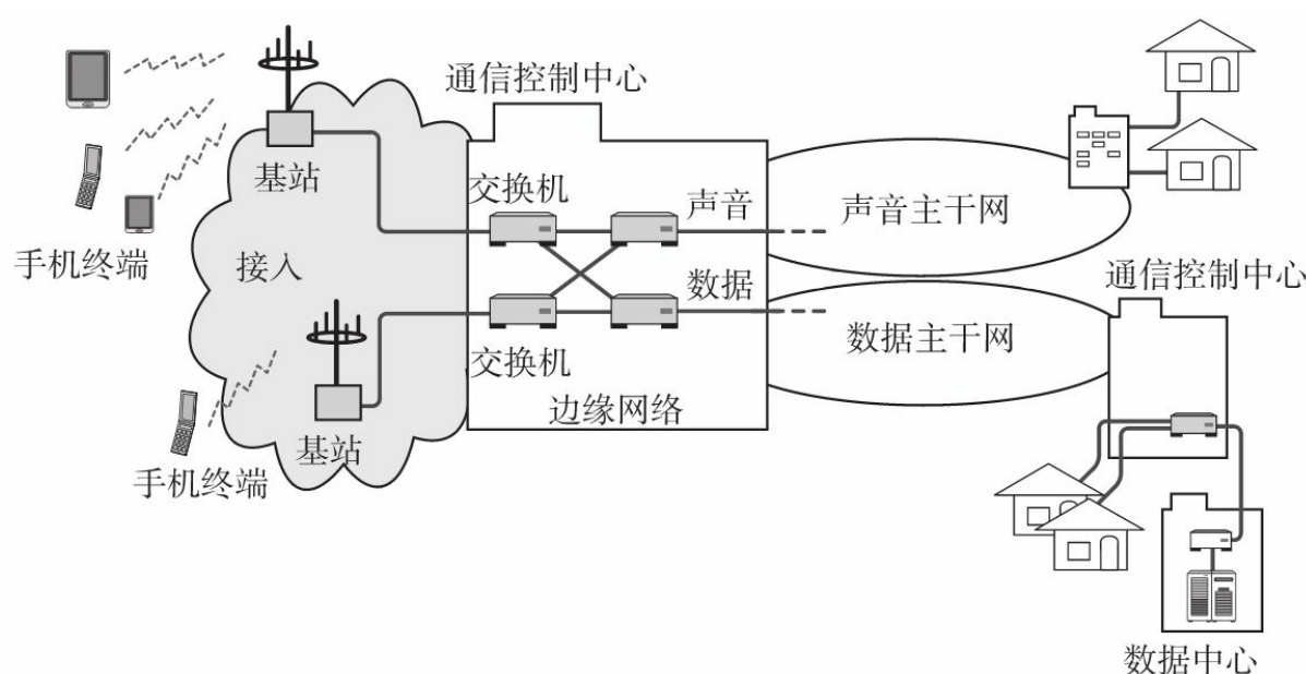
图1.53 移动通信
