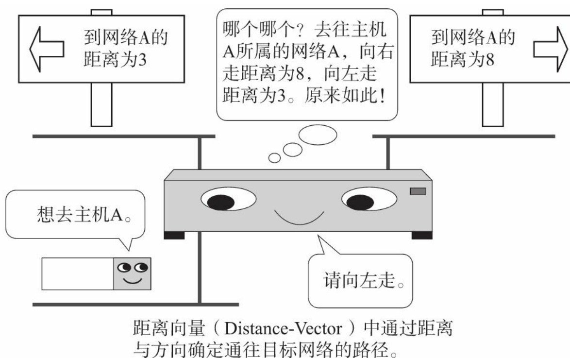
图7.4 距离向量
