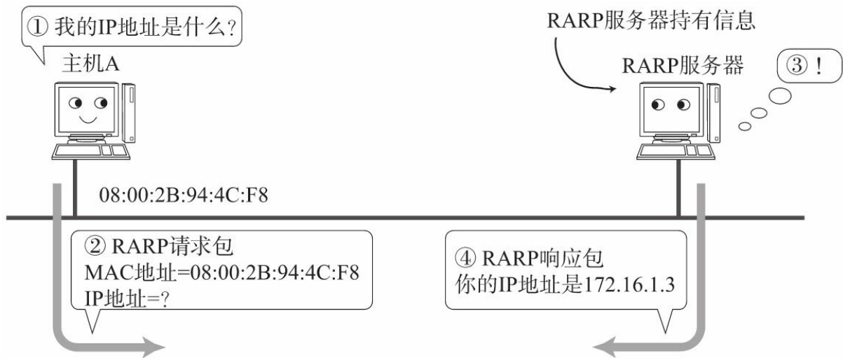
图5.9 RARP
