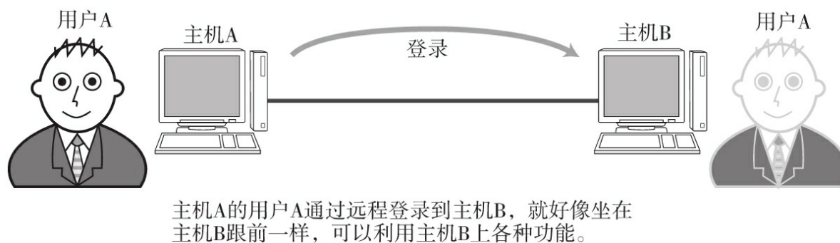
图8.2 远程登录
