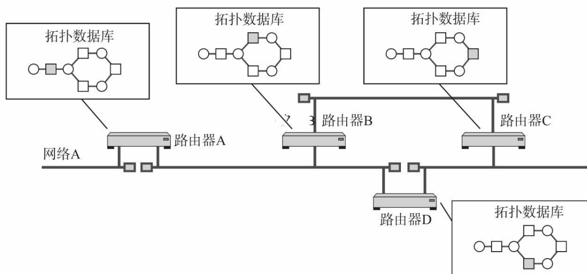
图7.13 由链路状态确定路由
