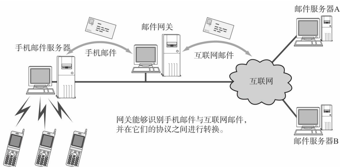
图1.47 手机与互联网电子邮件的转换
