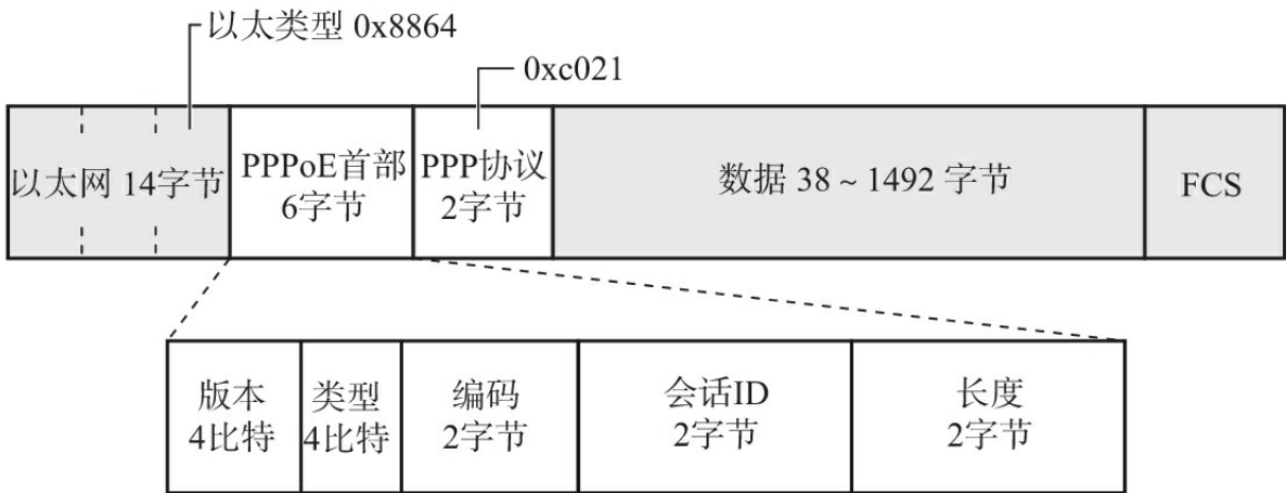
图3. 27 PPPoE数据帧格式
