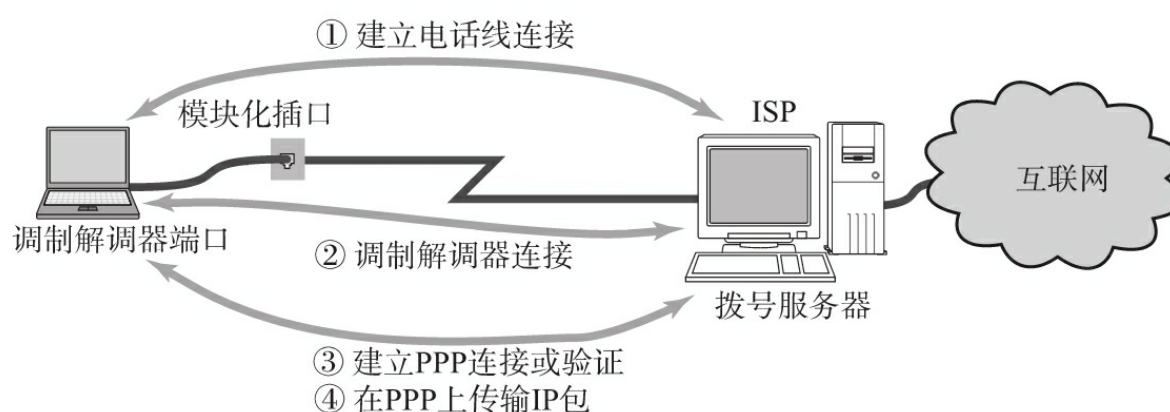
图3.25 PPP中建立连接
