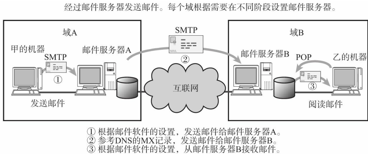
图8.10 现在互联网中电子邮件的发送过程
