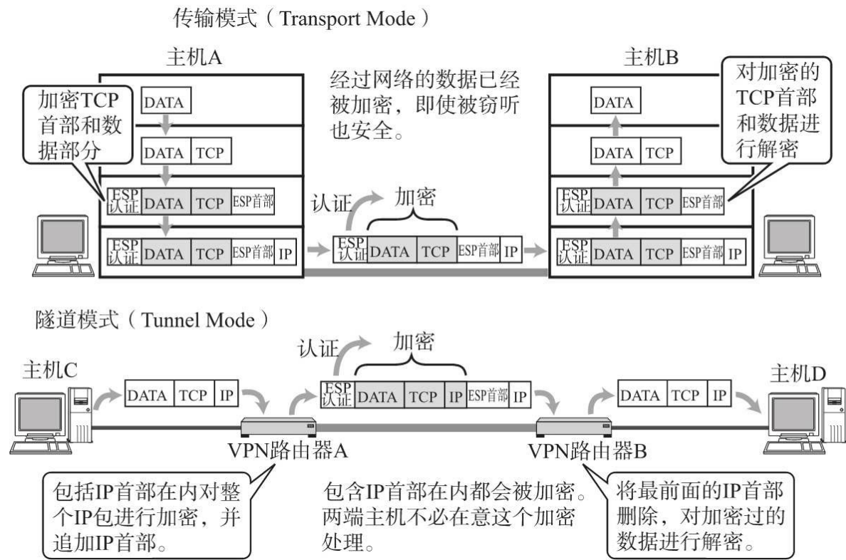
图9.7 通过IPsec加密IP包
