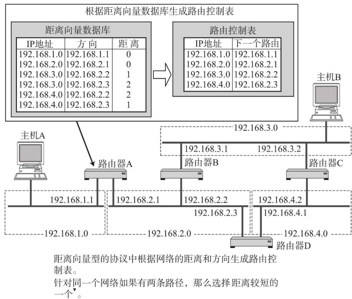
图7.7 根据距离向量生成路由控制表
