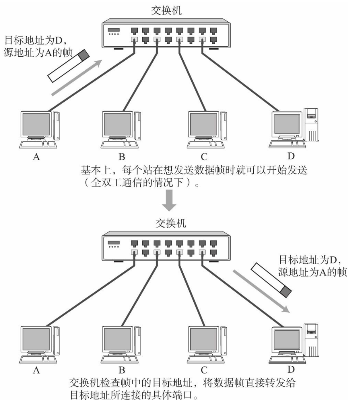
图3.9 非共享介质型网络
