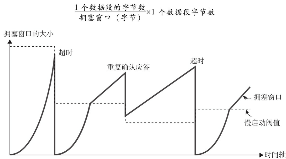
图6.21 TCP的窗口变化
