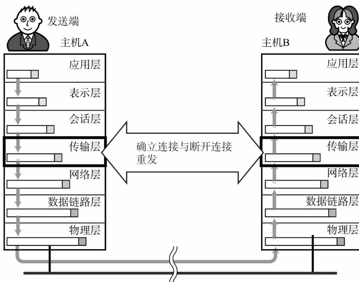
图1.25 传输层的工作
