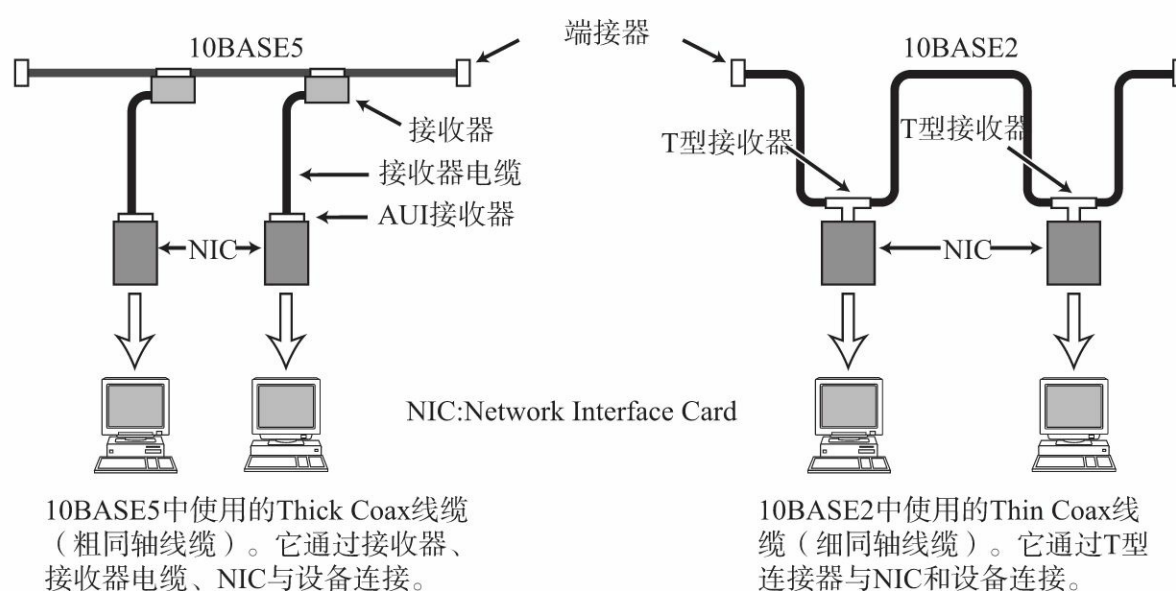
附图.6 10BASE5与10BASE2的网络构成
