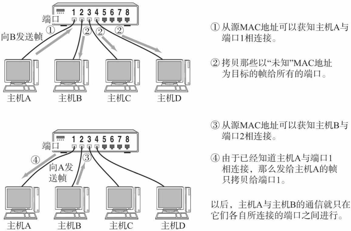
图3.12 交换机的自学原理
