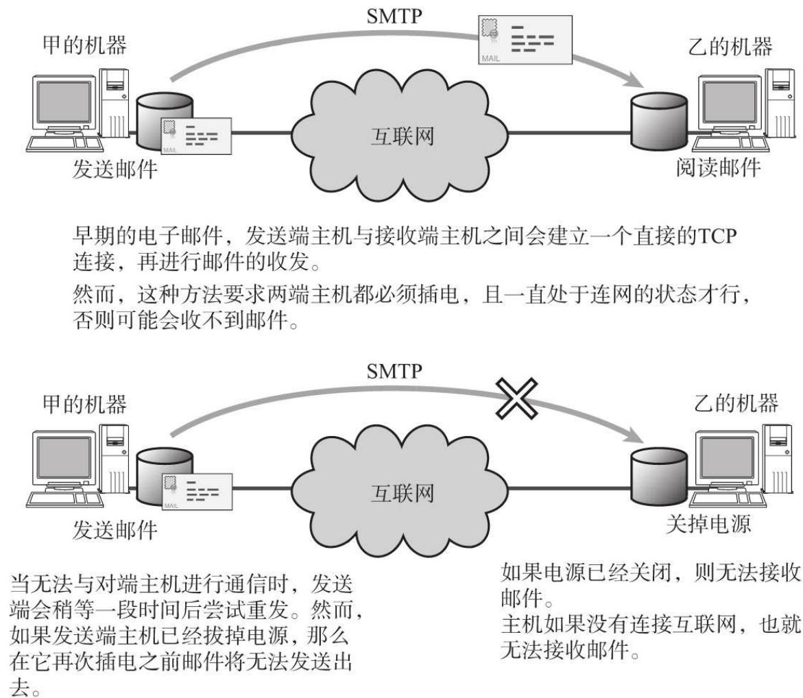
图8.9 早期的电子邮件发送过程
