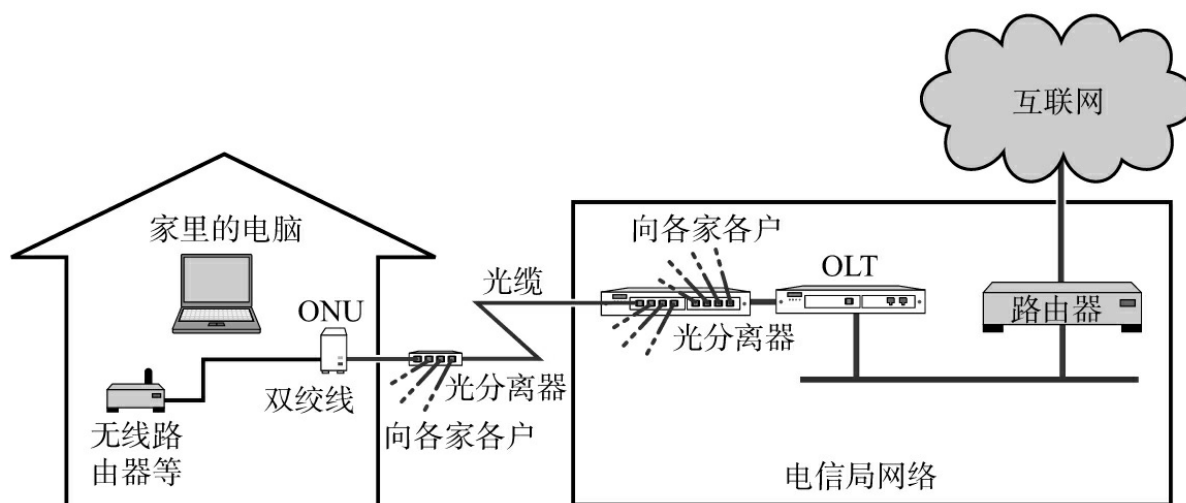
图3.35 FTTH连接
