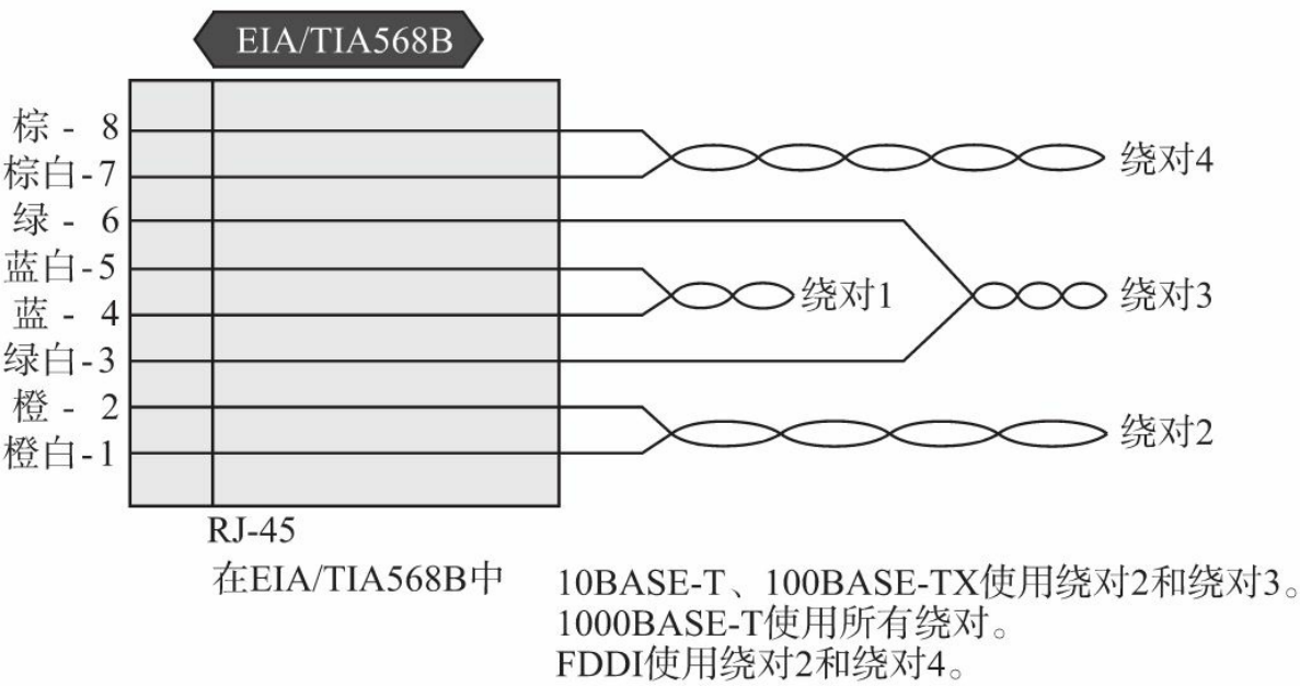
附图.9 双绞线绕对的组合方式
