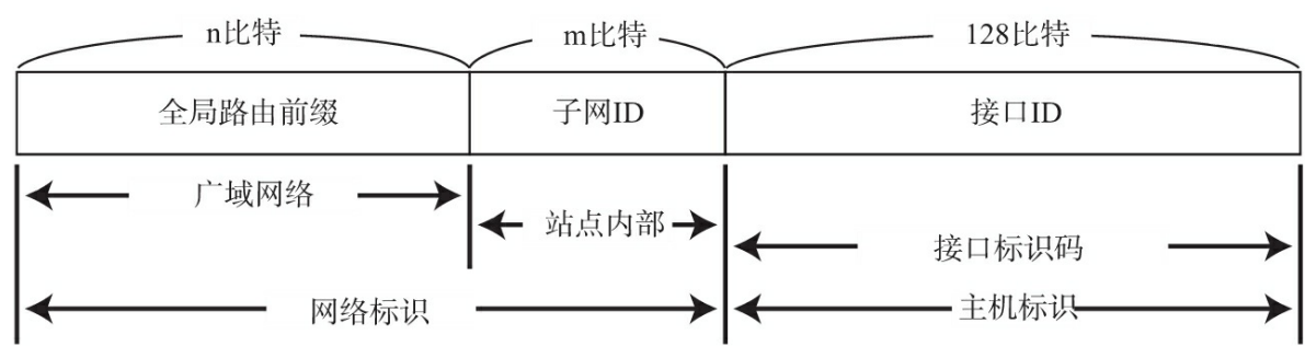
图4.28 全局单播地址
