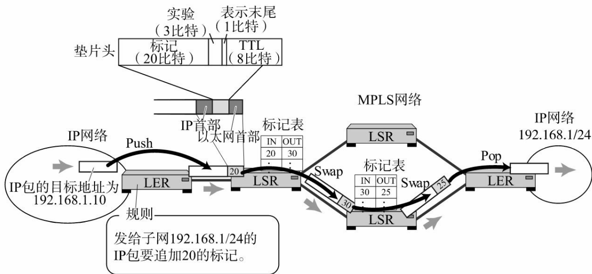
图7.23 使用Push、Swap和Pop功能进行转发
