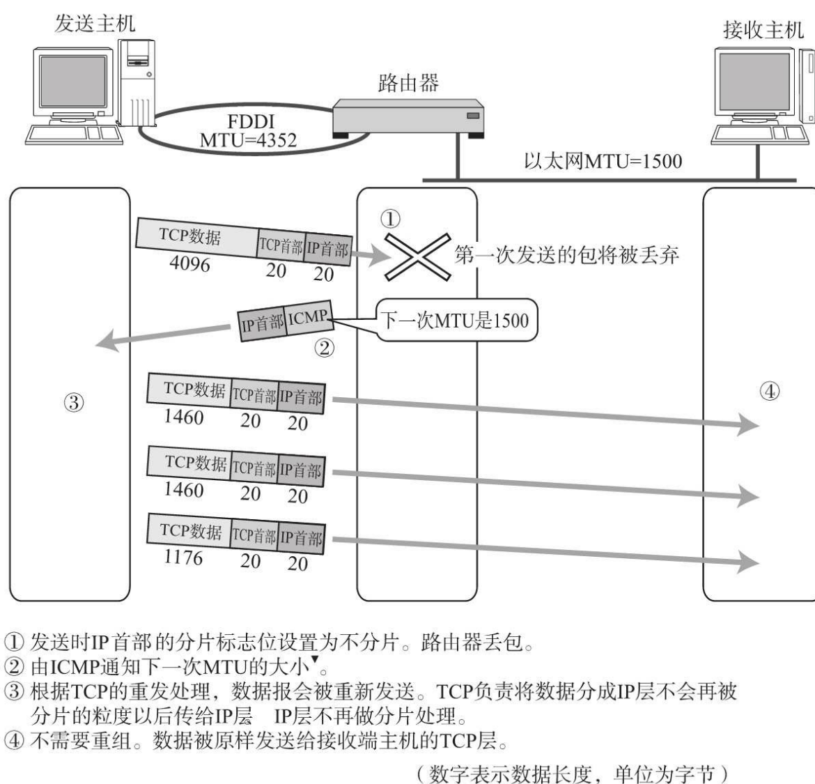
图4.26 路径MTU发现的机制 (TCP的情况下)
