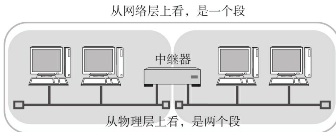
图3.2 段的范围
