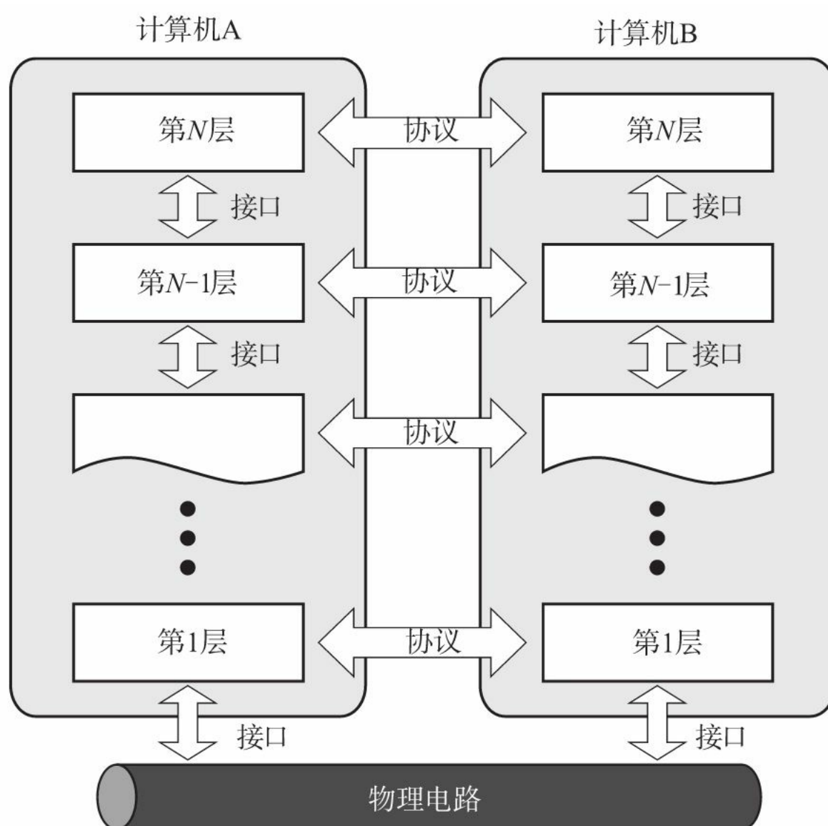
图1.16 协议的分层
