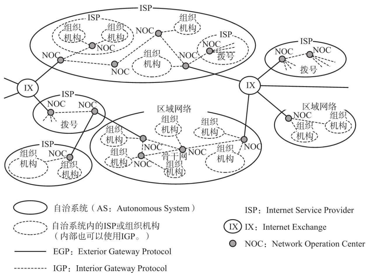
图7.3 EGP与IGP
