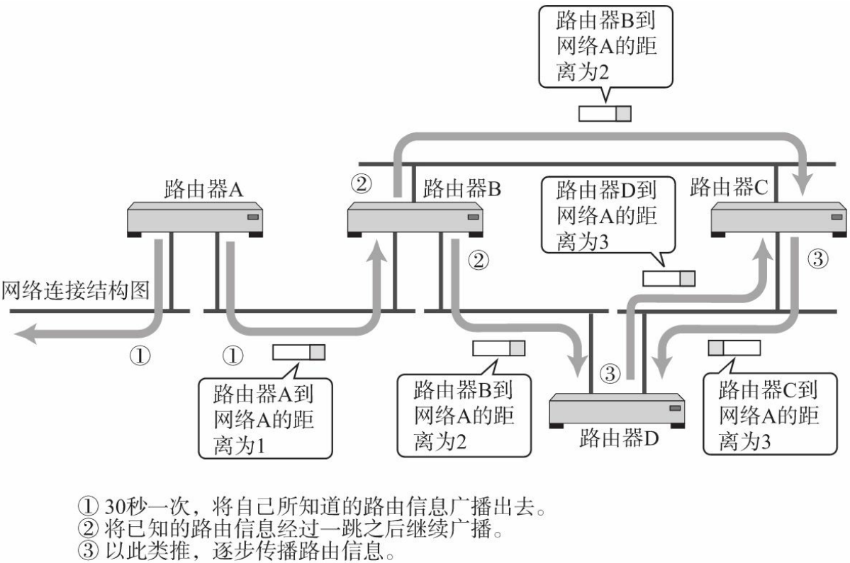
图7.6 RIP概要
