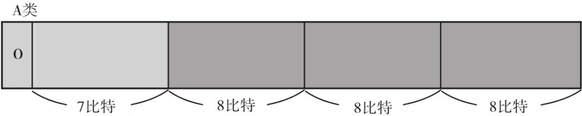
附图.1 A类
