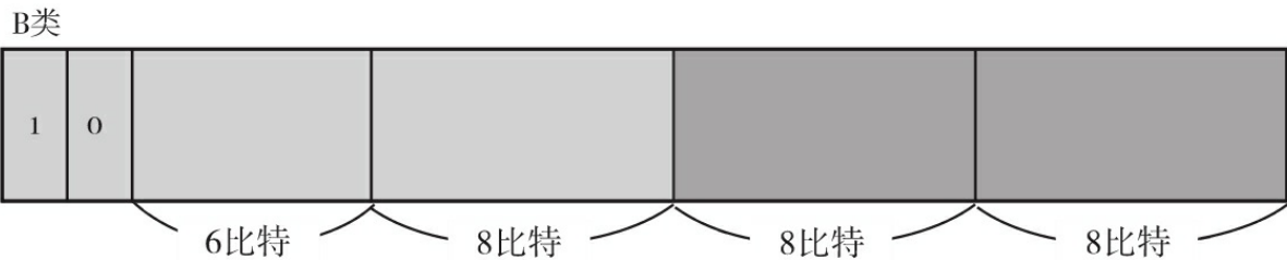
附图.2 B类
