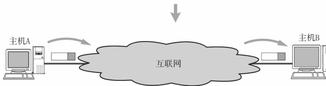
图2.9 互联网层
