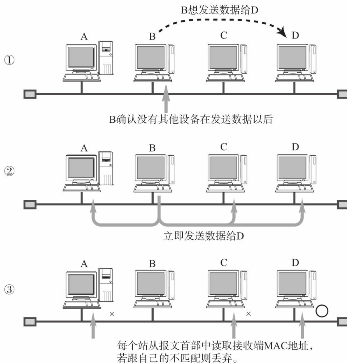
图3.6 争用方式
