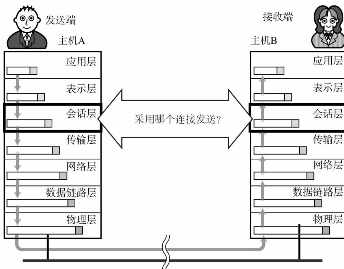
图1.24 会话层工作
