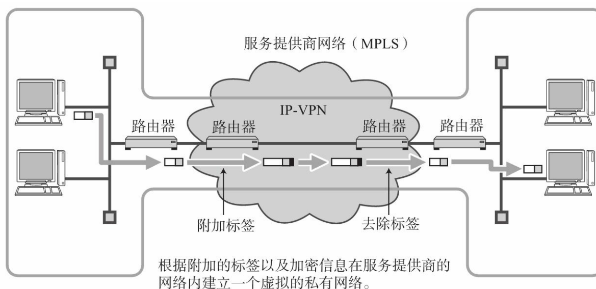
图3.37 IP-VPN（MPLS）
