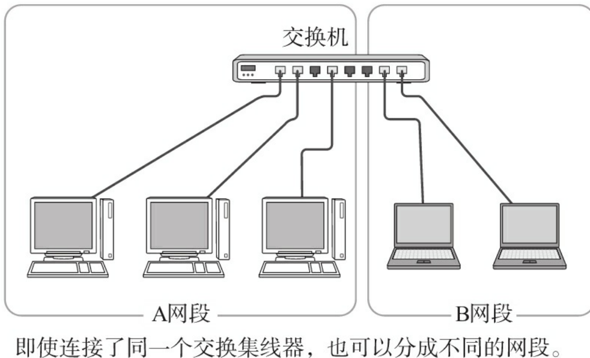
图3.15 简单的VLAN
