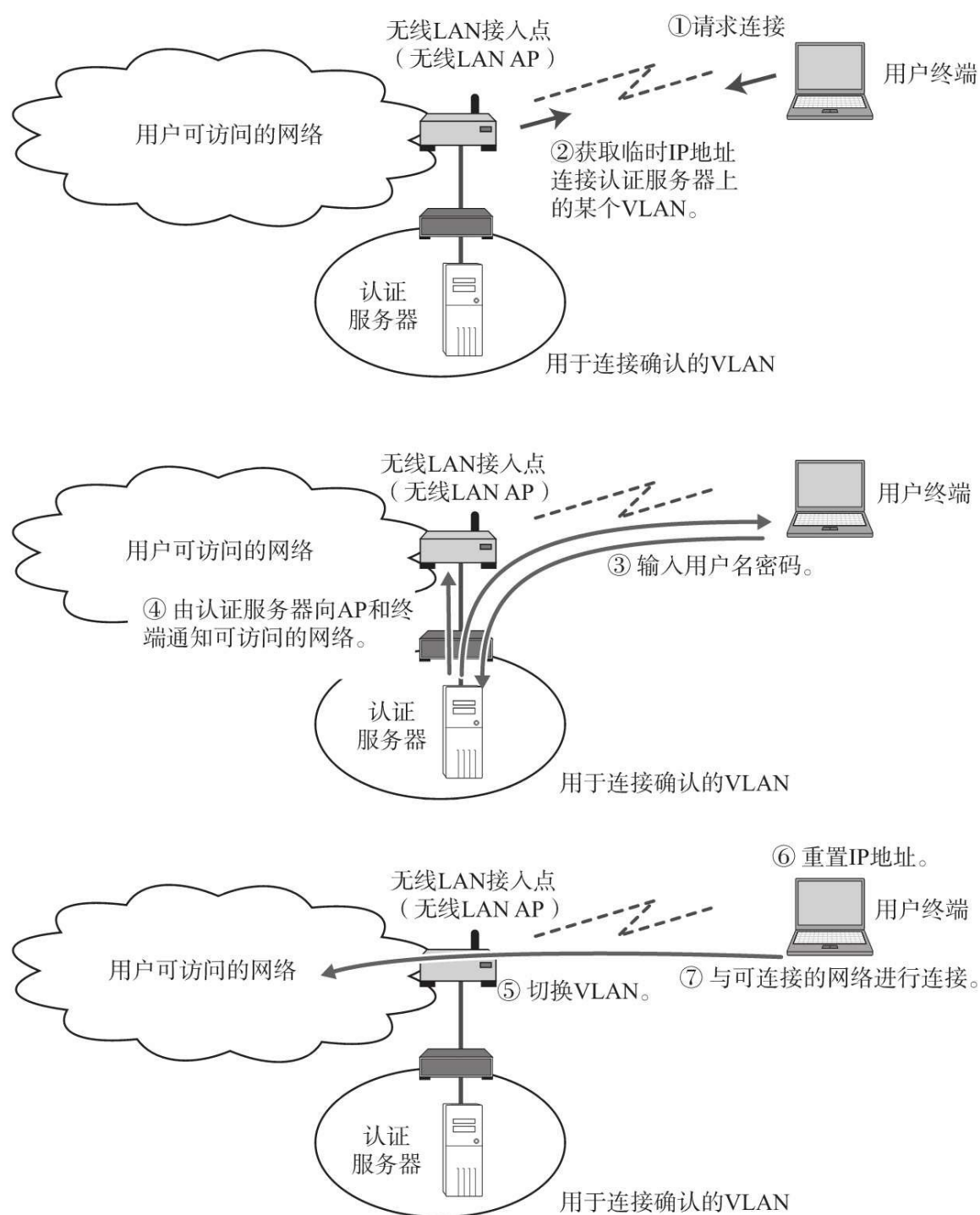
图9.9 IEEE802.1X
