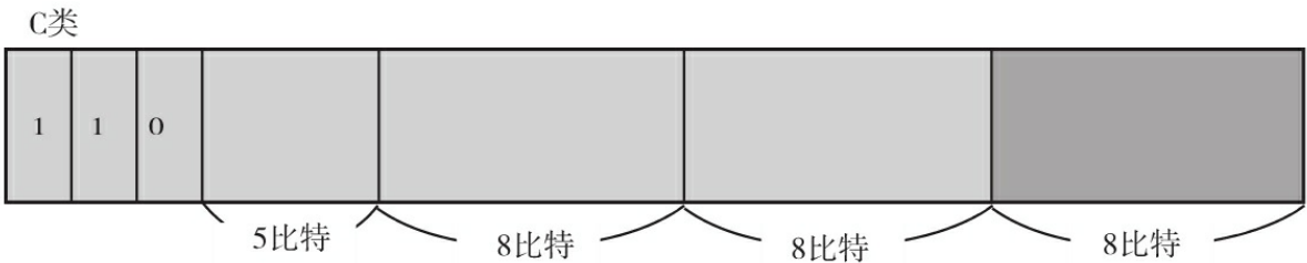
附图. 3 C类
