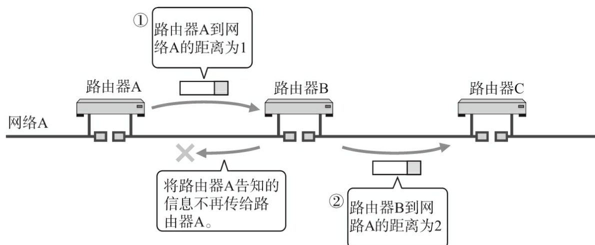
图7.10 水平分割
