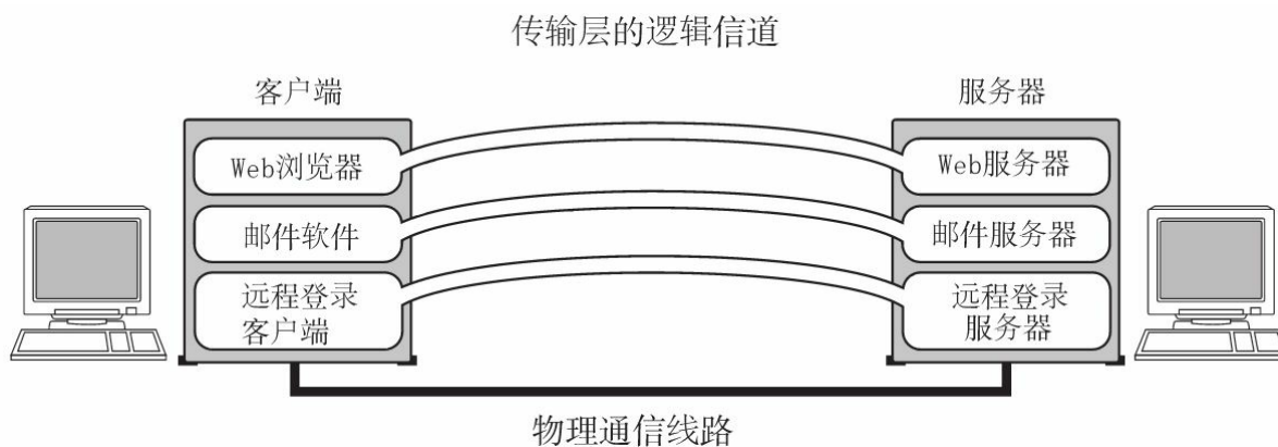
图2.10 传输层
