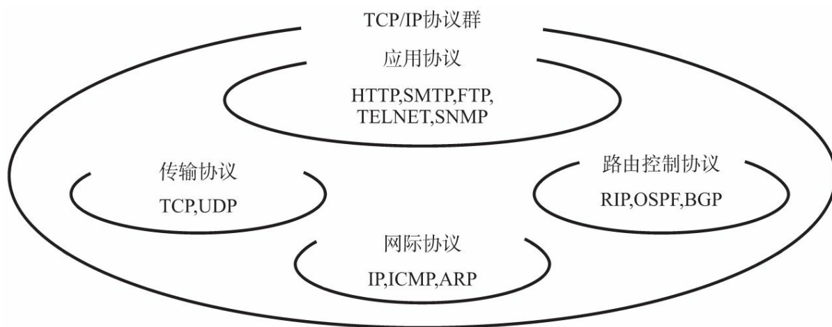
图2.3 TCP/IP协议群
