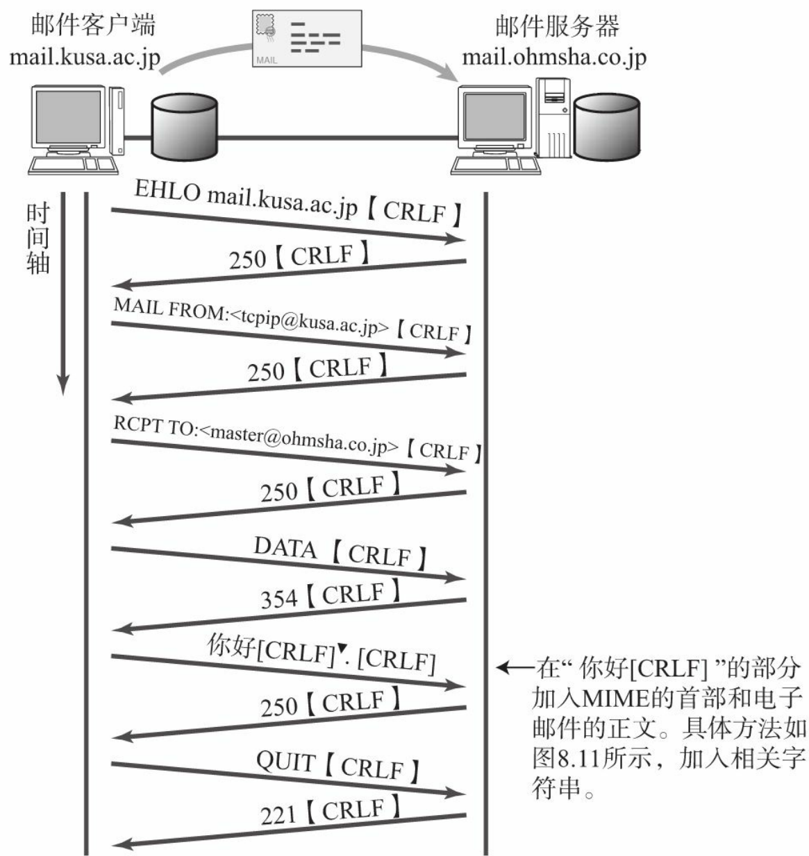
图8.12 SMTP
