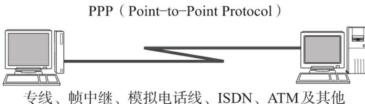
图3.24 PPP
