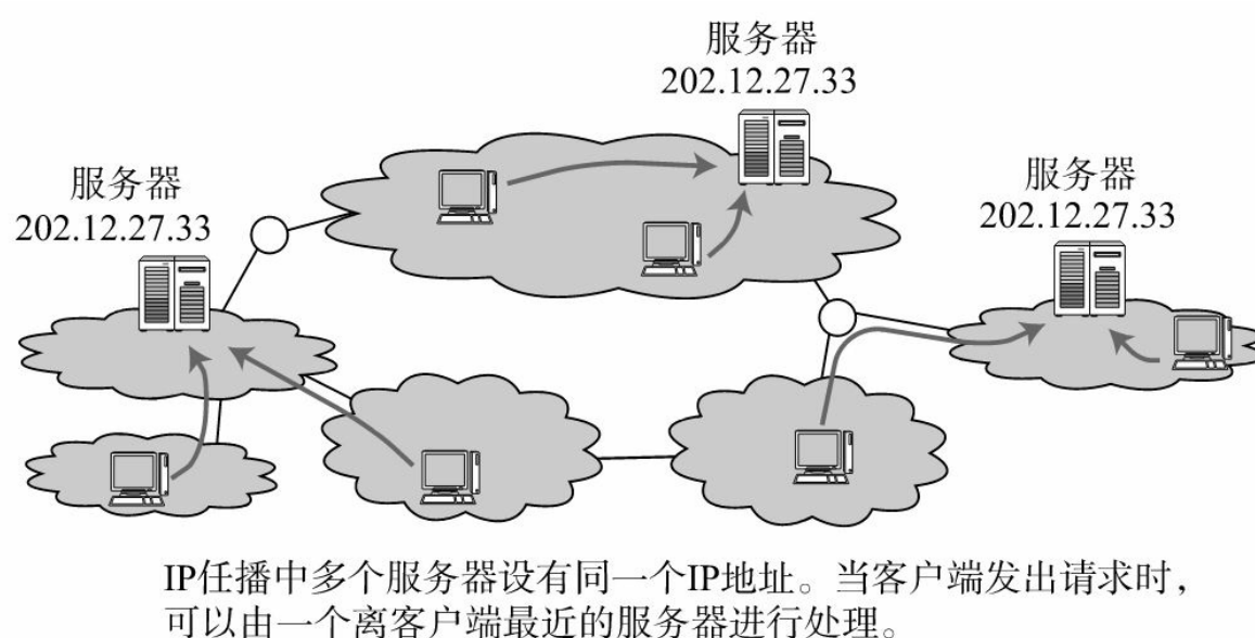
图5.26 IP任播
