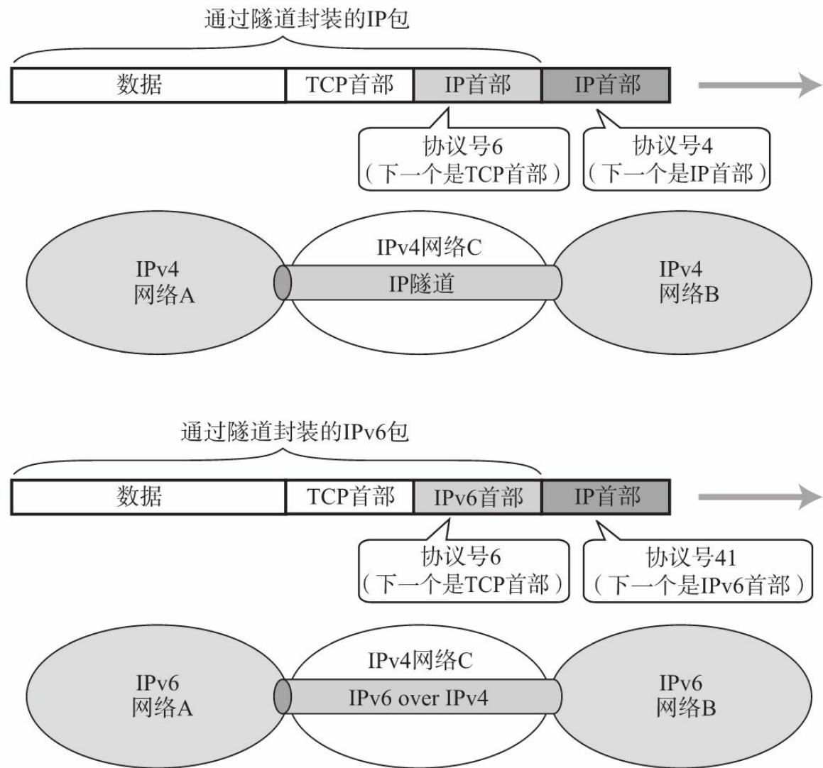
图5.23 IP隧道
