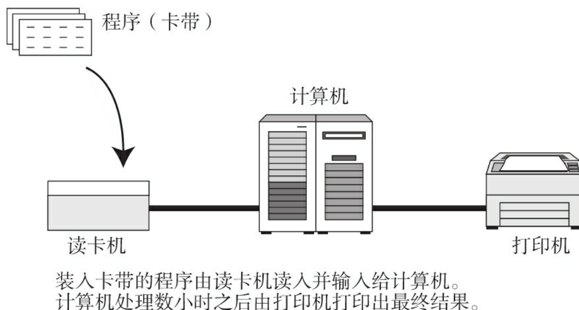
图1.5 批处理
