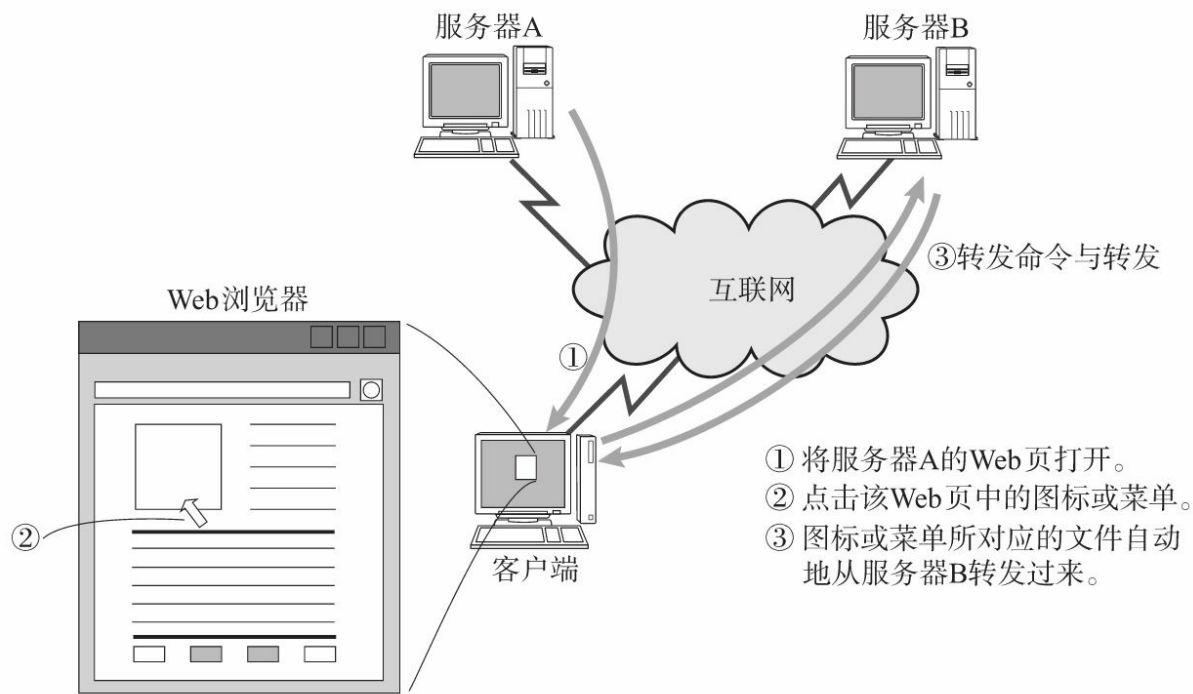
图8.15 WWW
