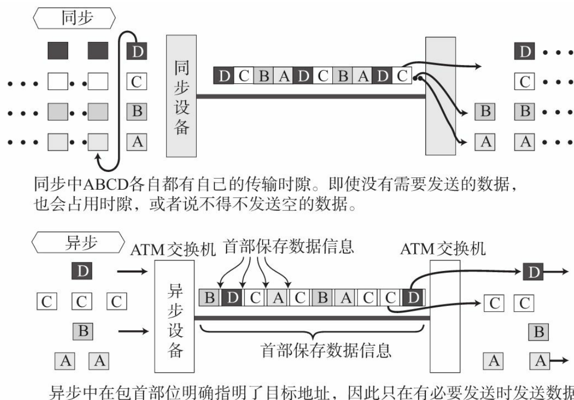
图3.29 同步与异步
