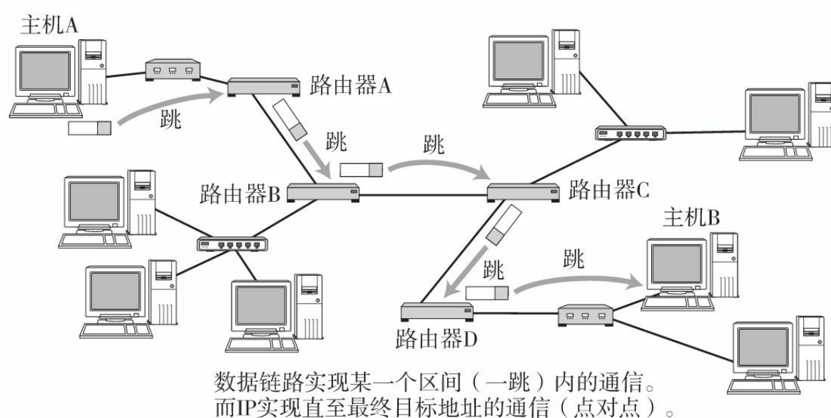
图4.5 多跳路由
