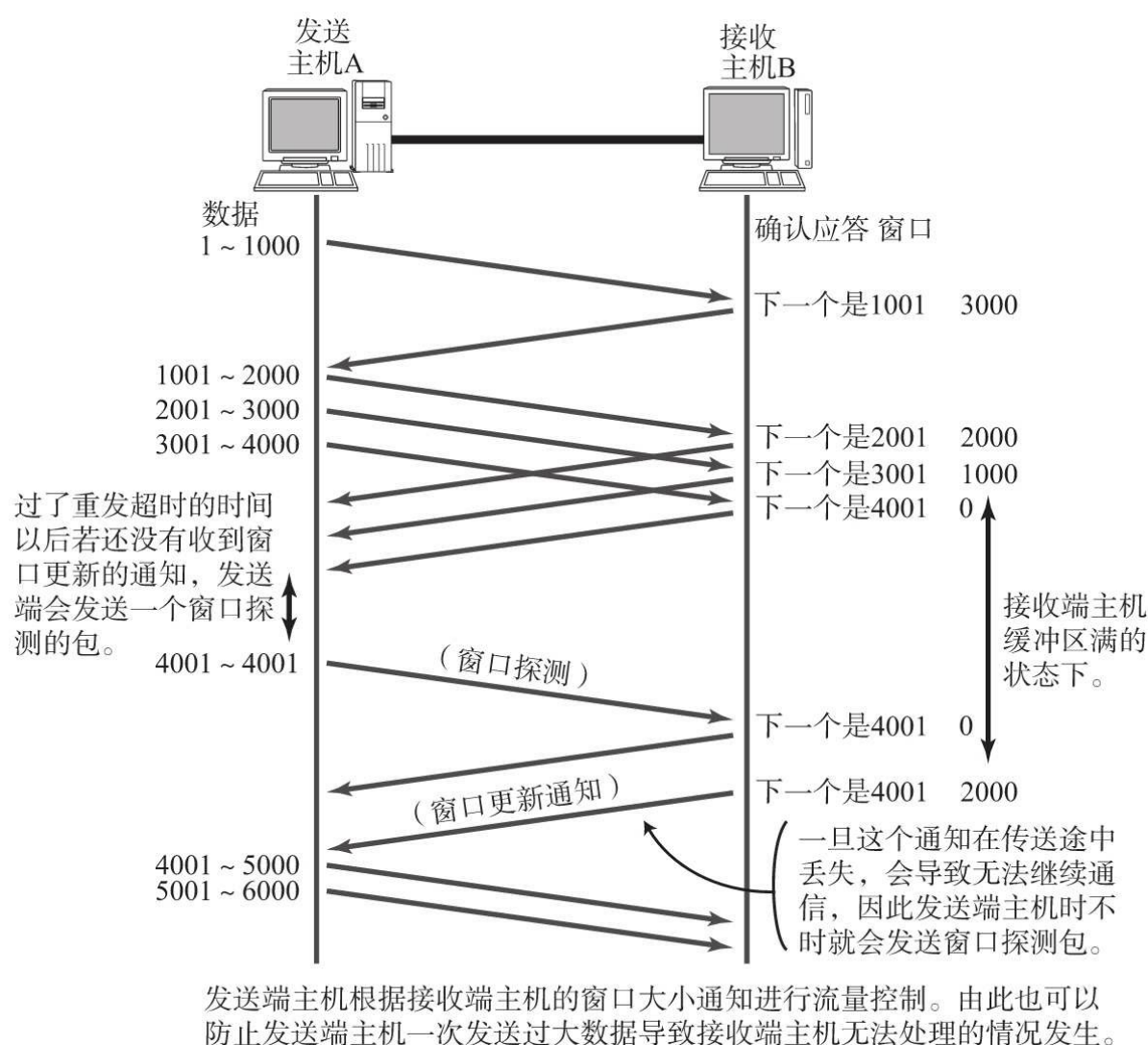
图6.19 流控制
