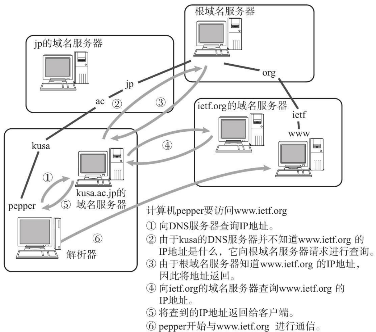
图5.5 DNS查询
