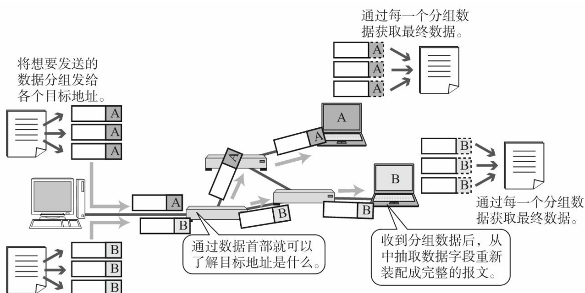
图1.30 分组交换
