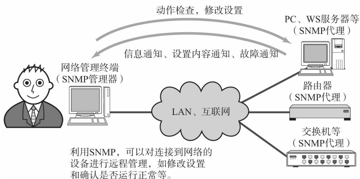
图8.20 网络管理
