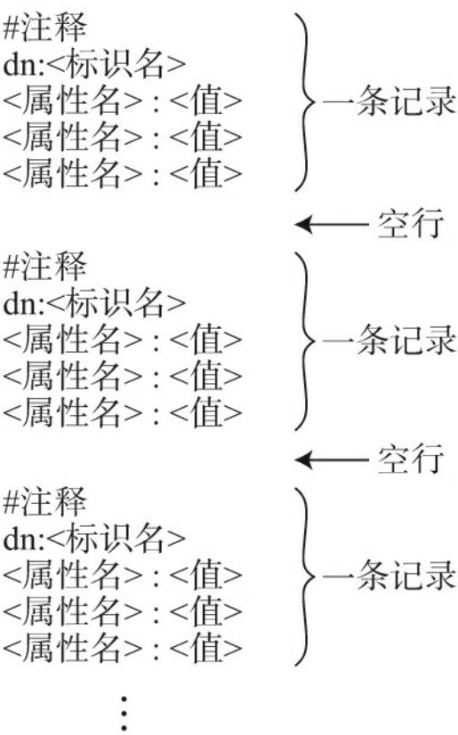
图8.29 LDIF文件
