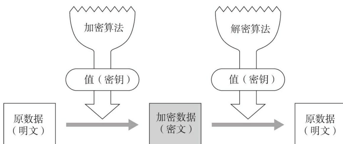
图9.4 加密过程
