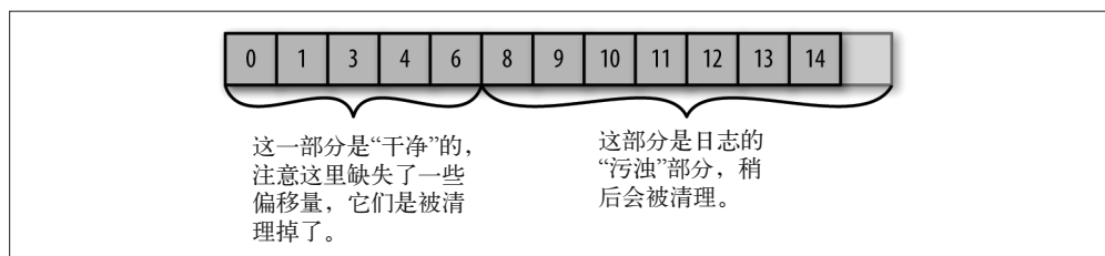
图 5-7：包含干净和污浊两个部分的分区
