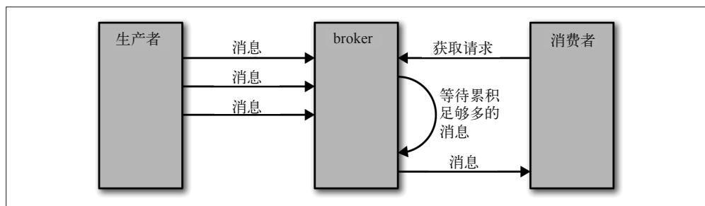
图 5-3: broker 延迟作出响应以便累积足够的数据
