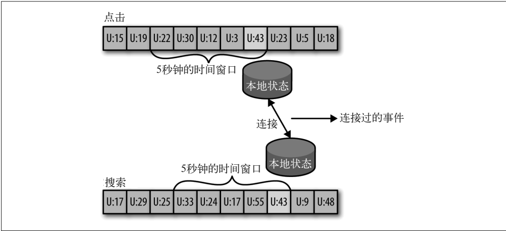
图 11-8：连接两个流，通常包含一个移动时间窗
