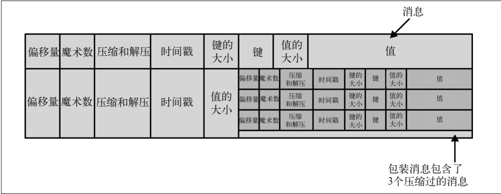
图 5-6：普通消息和包装消息
